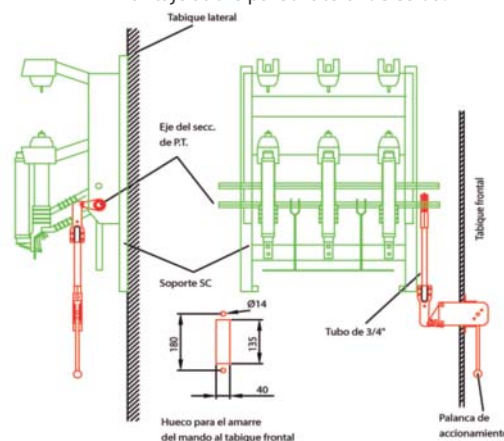
Montaje sobre pared lateral de celda:
