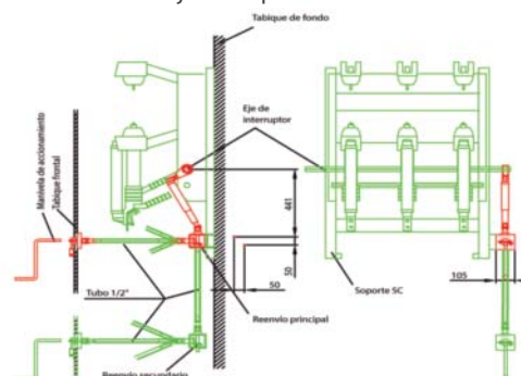
Montaje sobre pared de fondo de celda:
