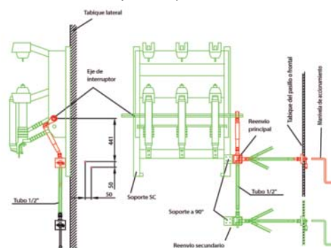
Montaje sobre pared lateral de celda:
