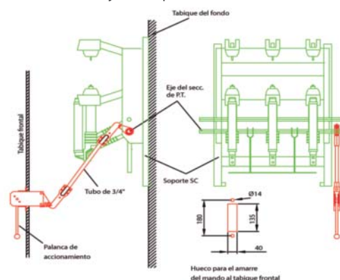
Montaje sobre pared de fondo de celda:
